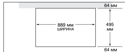
ВЫРЕЗ СТОЛЕШНИЦЫ
