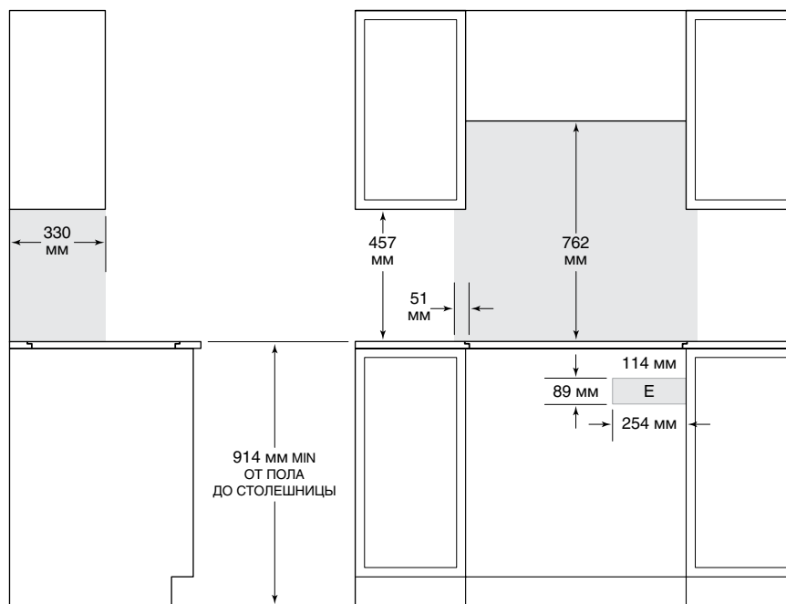
ВИД СБОКУ
