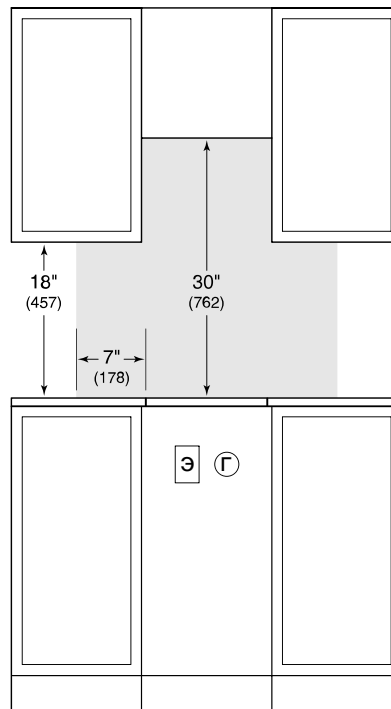
ВИД СПЕРЕДИ
